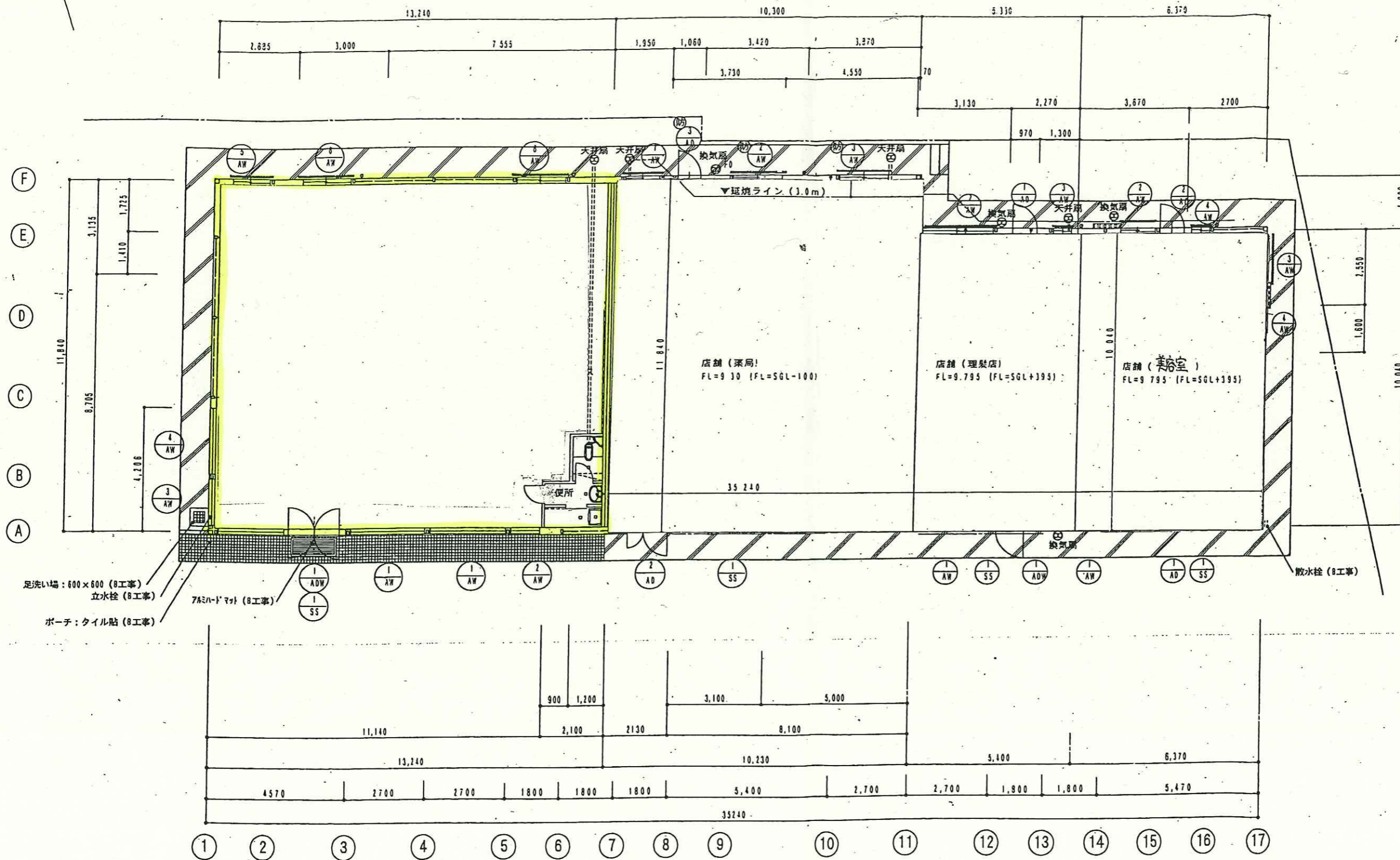
平面図 S:1/100
